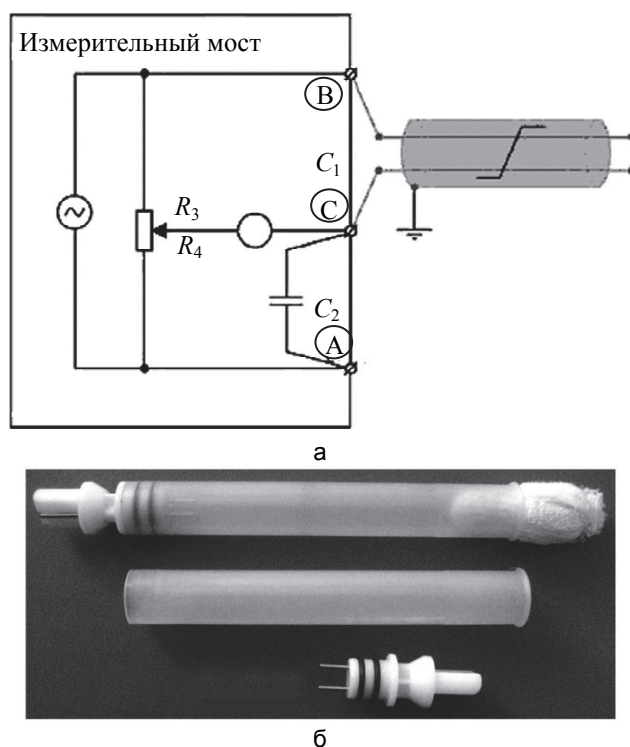
Рис. 1. Схема измерения импеданса (а) и устройство измерительной ячейки биоанализатора «Rabit» (со стерильно-марлевой пробкой и в разобранном виде) (б)
