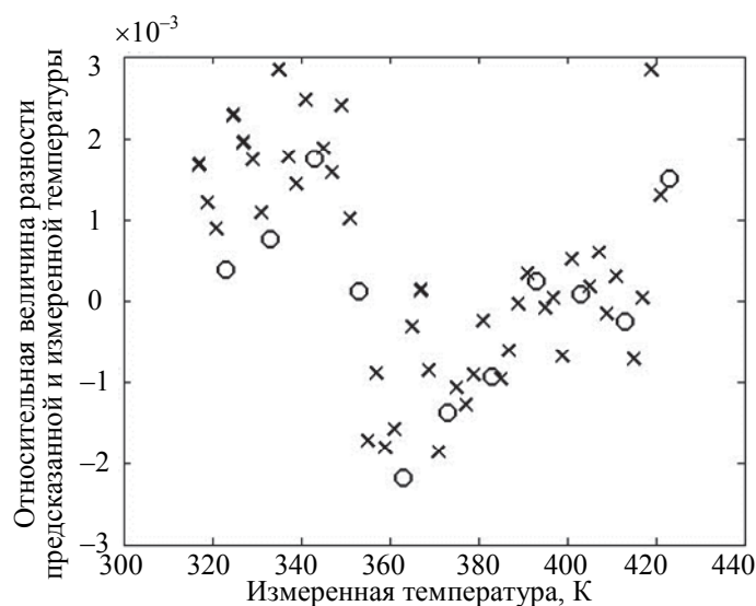
Рис. 4. Относительная разность между предсказанной методом FIR и измеренной температурой в зависимости от последней (кругами обозначены измерения, соответствующие спектрам, использованном для построения аппроксимации, крестиками – результаты аппроксимации)
