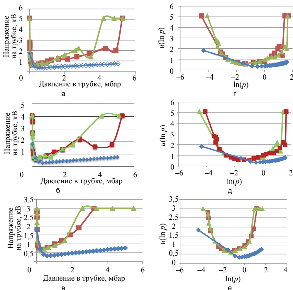
Рис. 2. Результаты измерений зависимости падения напряжения на разрядном промежутке от величины питающего разрядную цепь напряжения и давления воздушной смеси в разрядном промежутке в случаях откачки трубки (треугольные маркеры) и при напуске воздушной смеси (маркеры в виде квадратов) совместно с результатами численного моделирования в рамках полуэмпирического подхода для модельного газа (маркеры в виде ромбов).
