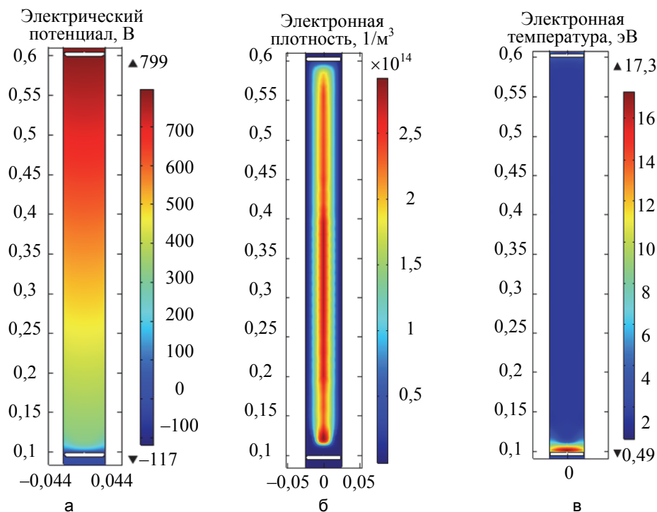
Рис. 10. Примеры двумерных распределений внутренних параметров разряда: электрического потенциала (а); концентрации (б), электронной температуры (в)
