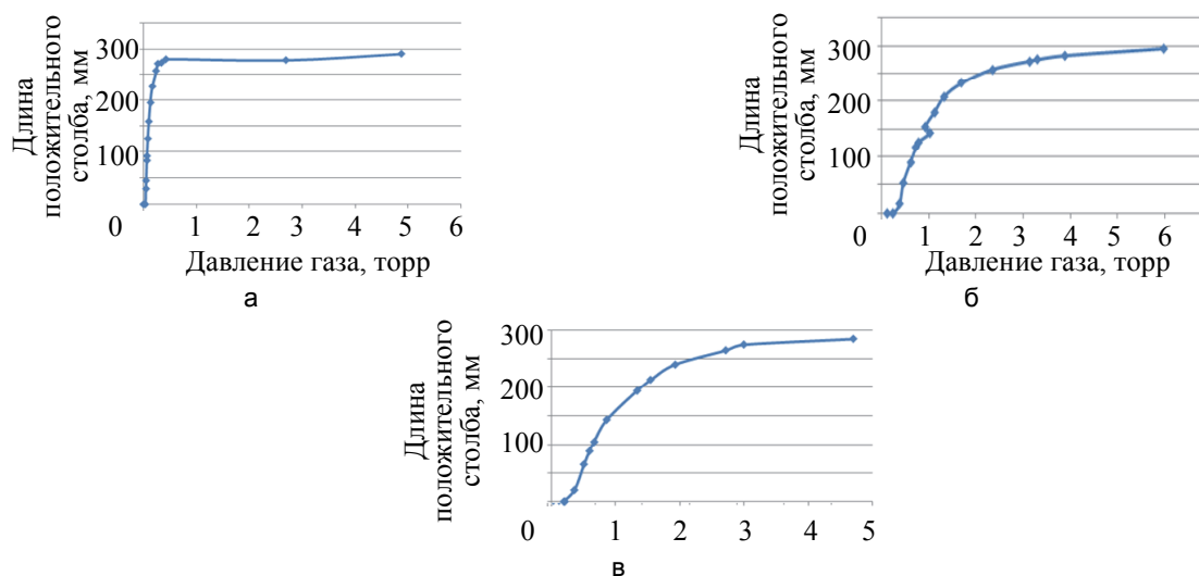
Рис. 3. Зависимость длины положительного столба тлеющего разряда в воздушной смеси от давления газа при различных значениях напряжений, питающих разрядную цепь: U=5,1 кВ (а); U=4,1 кВ (б); U=3,0 кВ (в)
