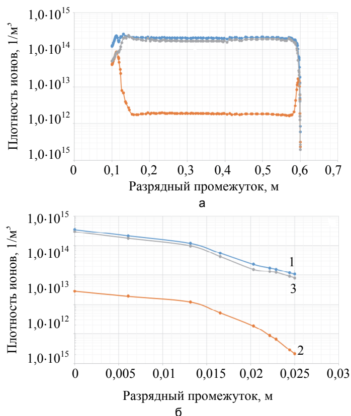
Рис. 6. Изменение продольных (а) и поперечных (б) профилей концентрации ионов основной компоненты воздушной смеси ( N_2 ) при учете элементарных процессов с участием кислорода: кривые 1 – концентрации N_2^+ в разряде в чистом азоте; кривые 2 – концентрации N_2^+ в разряде в воздухоподобной смеси с 30% добавкой кислорода; кривые 3 – концентрации O_2^+ в разряде в воздухоподобной смеси
