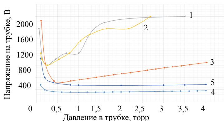
Рис. 4. Сопоставление результатов измерений электрических параметров тлеющего разряда в воздушной смеси (1 – при напуске газа, 2 – при откачке) с результатами, полученными в рамках полуаналитической модели (3) и численных гидродинамических микромоделей разряда в аргоне (4) и модельном одноатомном газе (5)
