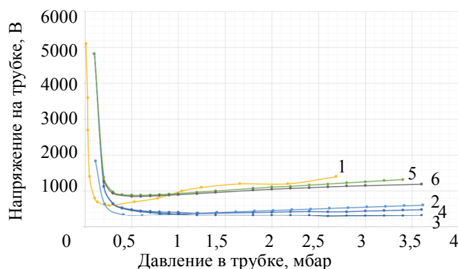
Рис. 5. Результаты расчетов зависимости от давления величины падения напряжения на разрядном промежутке для различных плазмохимических моделей нелокальной плазмы: 1 – эксперимент; 2 – полуаналитическая модель; 3 – учет в рамках гидродинамической модели совокупности реакций (3); 4 – учет реакций (3) совместно с возбуждением колебаний и вращений молекул (4); 5 – дополнительный учет неупругих столкновений (5), приводящий к электронному возбуждению молекул; 6 – модель, учитывающая всю совокупность процессов (3)–(6) для разряда в смеси азота и кислорода
