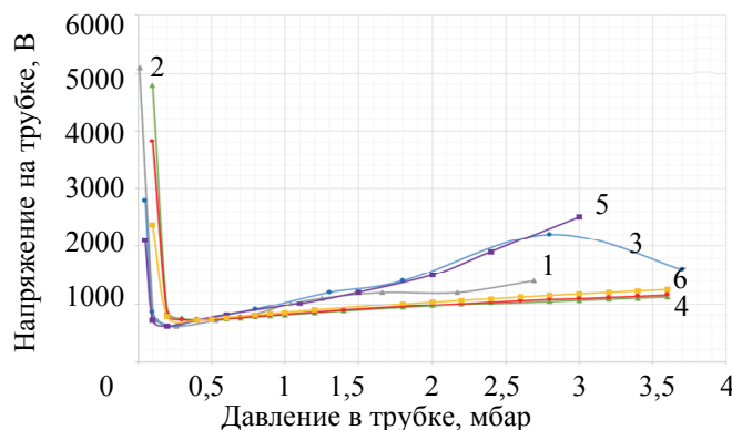
Рис. 8. Сопоставление экспериментально полученных зависимостей u(p) с результатами численного моделирования с учетом реакций (3)–(6) при уточненном значении \gamma = 0,02 : кривые 1 и 2 – эксперимент и результаты моделирования при U_1 = 5,1 кВ; кривые 3 и 4 – эксперимент и результаты моделирования при U_2 = 4,1 кВ; кривые 5 и 6 – эксперимент и результаты моделирования при U_3 = 3,0 кВ
