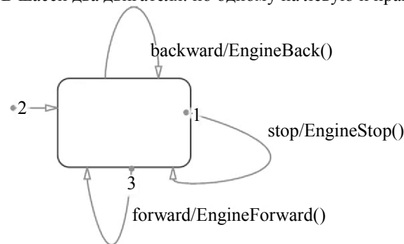
Рис. 1. Граф переходов автоматного типа AEngine
