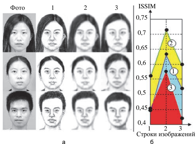
Рис. 5. Оценка ISSIM для вариантов «свой» или «чужой» скетч: три разных фотоизображения (база СУНК) и соответствующие им скетчи (колонка 1), результаты «размытия» скетчей (колонка 2) и скетчи, не соответствующие исходному изображению, также полученные в результате их «размытия» (колонка 3) (а); значения ISSIM между исходными фотоизображениями и тремя скетчами в соответствующей строке. По оси абсцисс отмечены номера строк скетчей, а по оси ординат – значения ISSIM. Цифрами в кружочке отмечены: 1 – кривая значений ISSIM для исходных скетчей; 2 – значения ISSIM для результата «размытия» этих скетчей (по определению выше – «своих скетчей») и 3 – значения ISSIM для результата «чужого скетча» (б)
