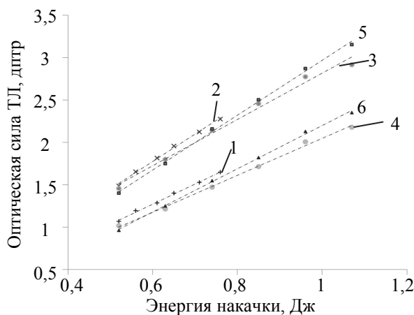
Рис. 5. Пересчитанные зависимости оптической силы тепловой линзы на длине волны 1,55 мкм в Yb-Er-стекле при диодной накачке в разных режимах: 1 – модуляция добротности ( \varphi -компонента), 2 – модуляция добротности ( \gamma -компонента), 3 – свободная генерация ( \gamma -компонента), 4 – свободная генерация ( \varphi -компонента), 5 – без генерации ( \gamma -компонента), 6 – без генерации ( \varphi -компонента)
