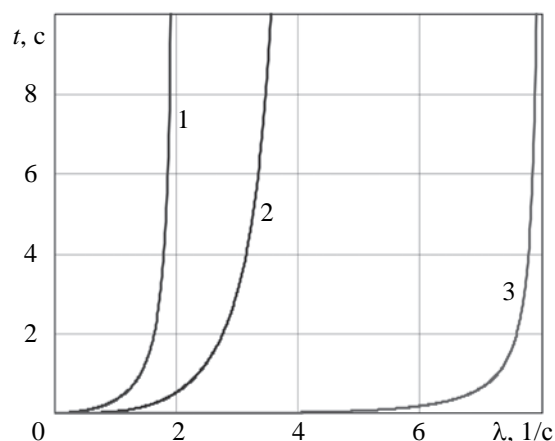
Рис. 1. Зависимость среднего времени ожидания от интенсивности поступления заявок \lambda . Кривые 1–3 соответствуют кратности резервирования запросов k = 4, 2, 1
