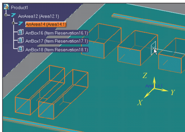
Рис. 3. Процесс выделения объема в «CATIA»(Plant Layout)
