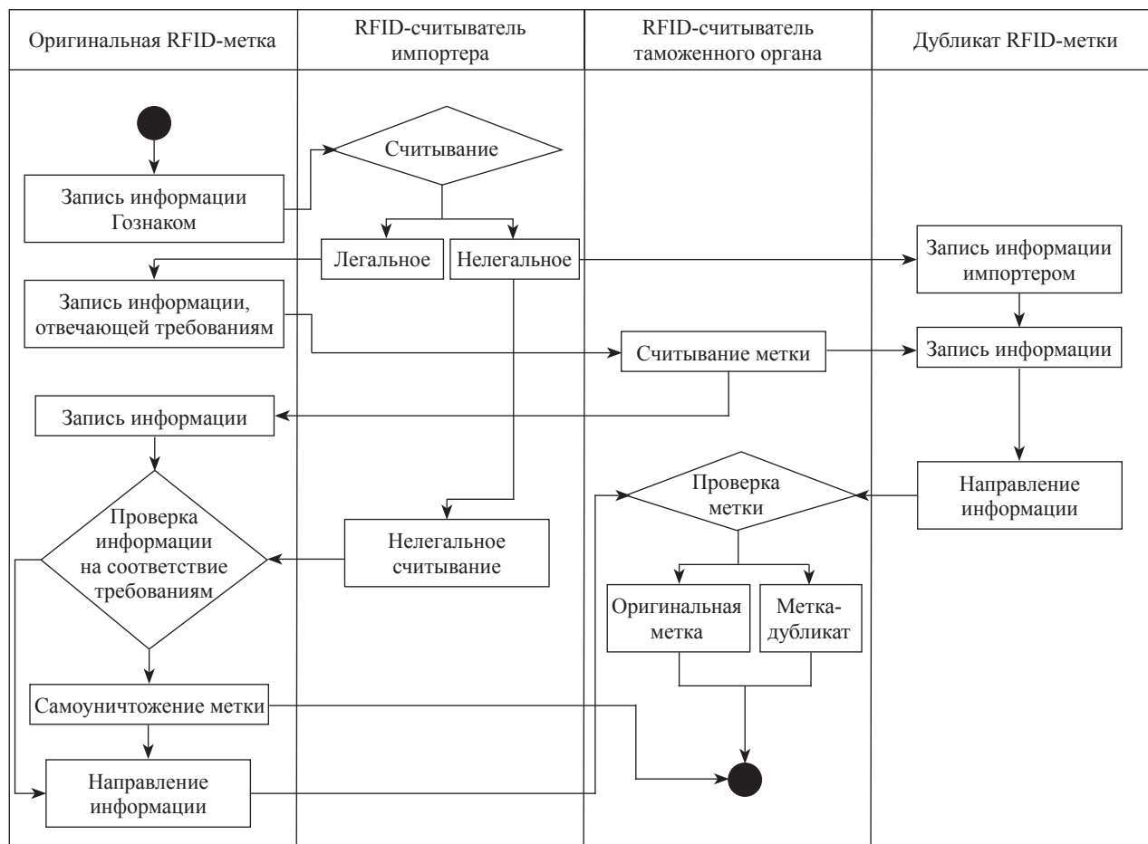
Рис. 2. Предлагаемый алгоритм обнаружения RFID-дубликатов Fig. 2. The proposed algorithm for detecting RFID duplicates
