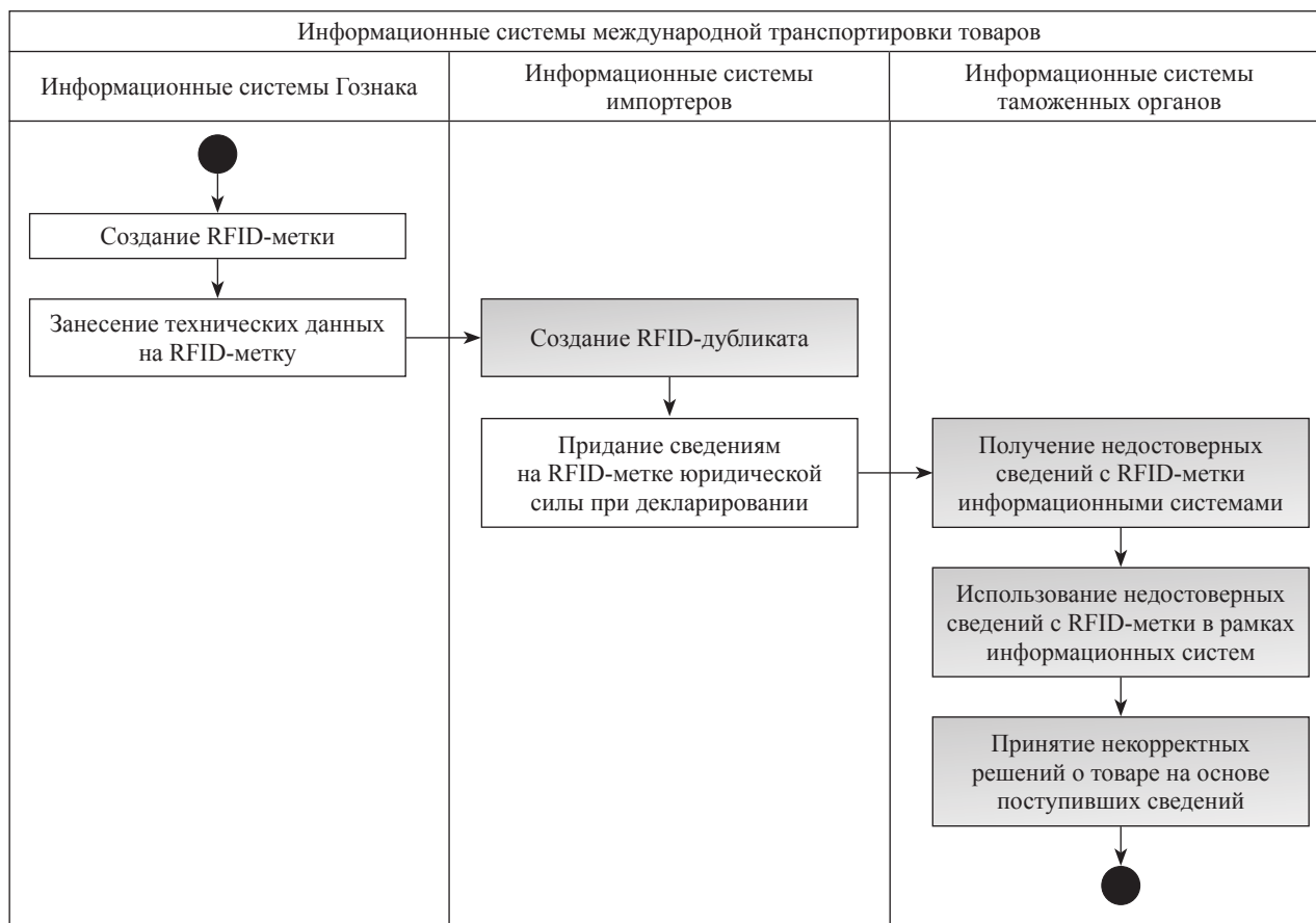
Рис. 1. Модель использования RFID-дубликатов для формирования искаженных сведений в информационных системах международной транспортировки товаров
