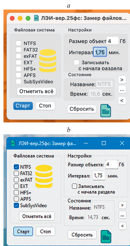
Рис. 4. Интерфейс приложения для измерения времени доступа к данным под MacOS (a) и Windows (b)
