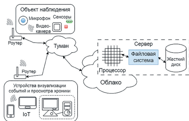
Рис. 1. Место файловой системы на видеосервере в интеллектуальной системе видеонаблюдения.
