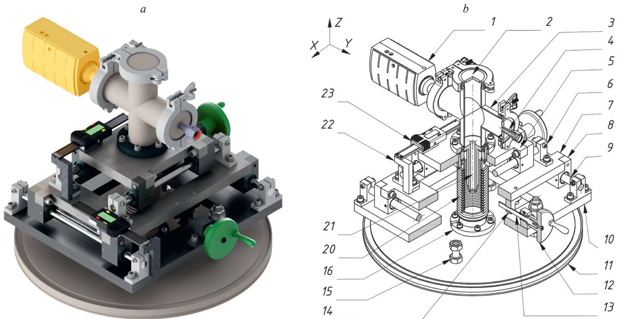
Рис. 1. Конструкция манипулятора: внешний вид (а) и схема (b).
