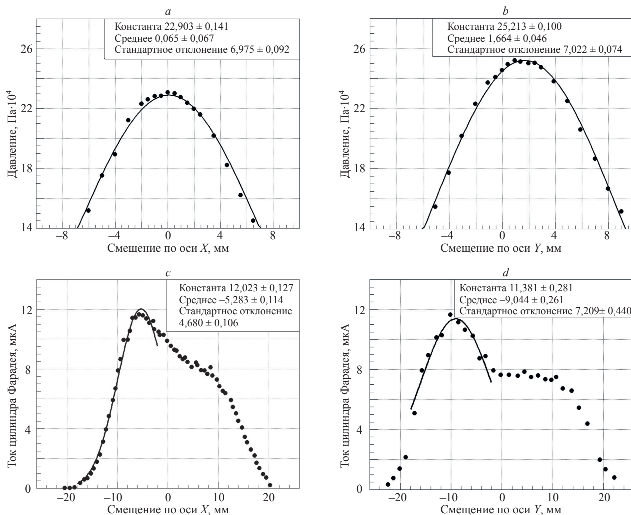
Рис. 3. Результаты измерений интенсивностей пучков атомов (a, b) и ионов (c, d) дейтерия, произведенных посредством компрессионной трубки (a, b) и цилиндра Фарадея (c, d) при прямолинейном их перемещении через геометрический центр вакуумного тракта атомарной и ионной ступеней источника POLIS: смещения вдоль оси X (a, c) и Y (b, d).
