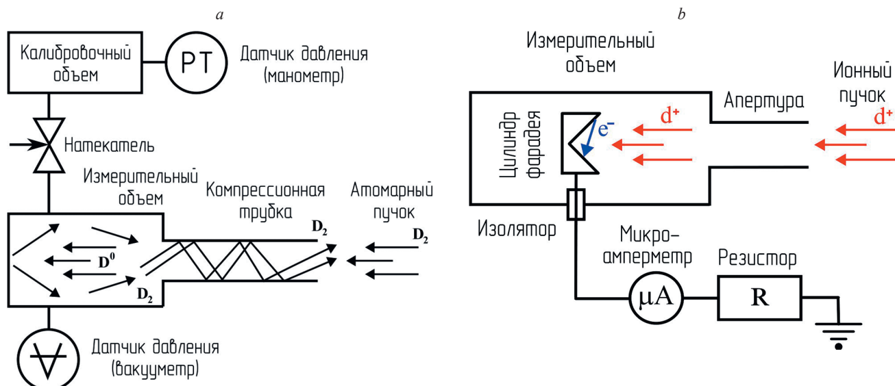
Рис. 2. Принципы действия устройств для измерения интенсивности ионного и атомарного пучков: компрессионная трубка для атомарного пучка (а); цилиндр Фарадея для ионного пучка (b).
