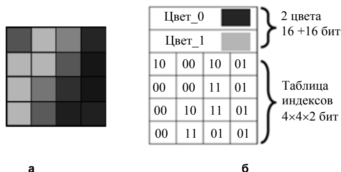
Рис. 1. Пример блока BC1: исходный блок 4×4 пикселя размером 512 бит (а); сжатый блок размером 64 бита (б)
