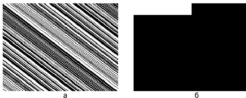
Рис. 6. Портрет матрицы M_{167} (а) и гистограмма модулей ее элементов (б)
